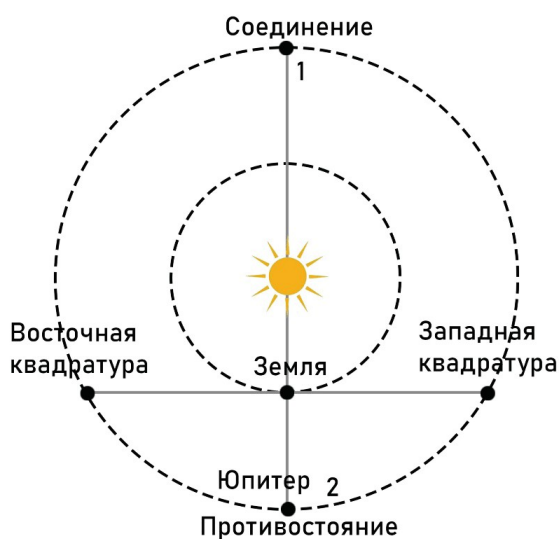
Рисунок 3-1. Особые точки орбиты внешних планет
