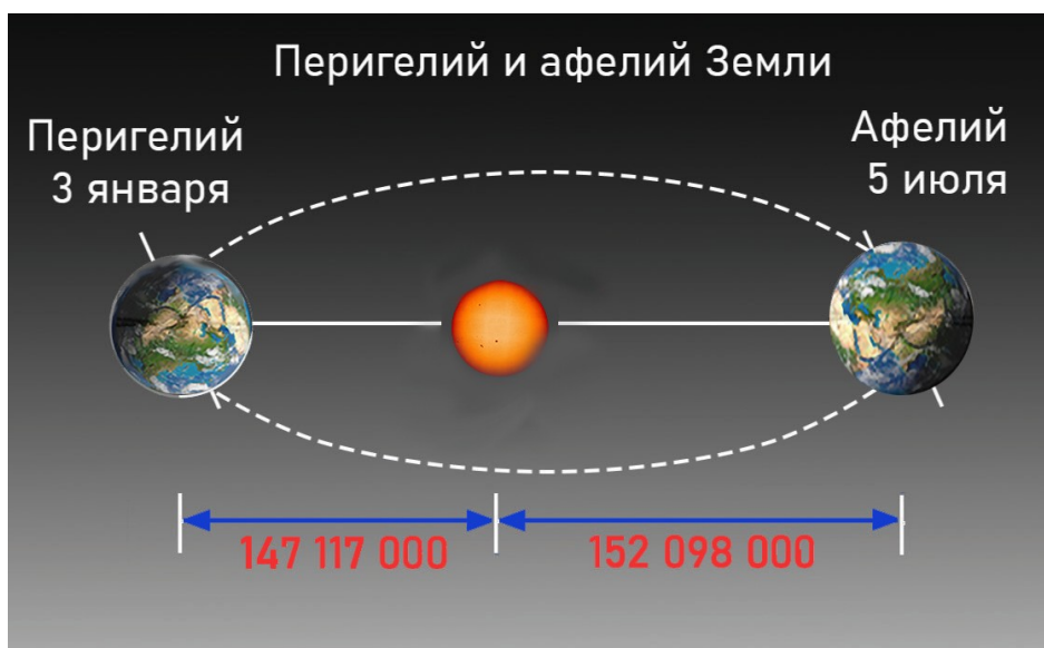
Рисунок 1-33. Изменение расстояния от Солнца зимой и летом
