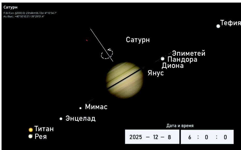
Рисунок 3-37. Сатурн без колец
