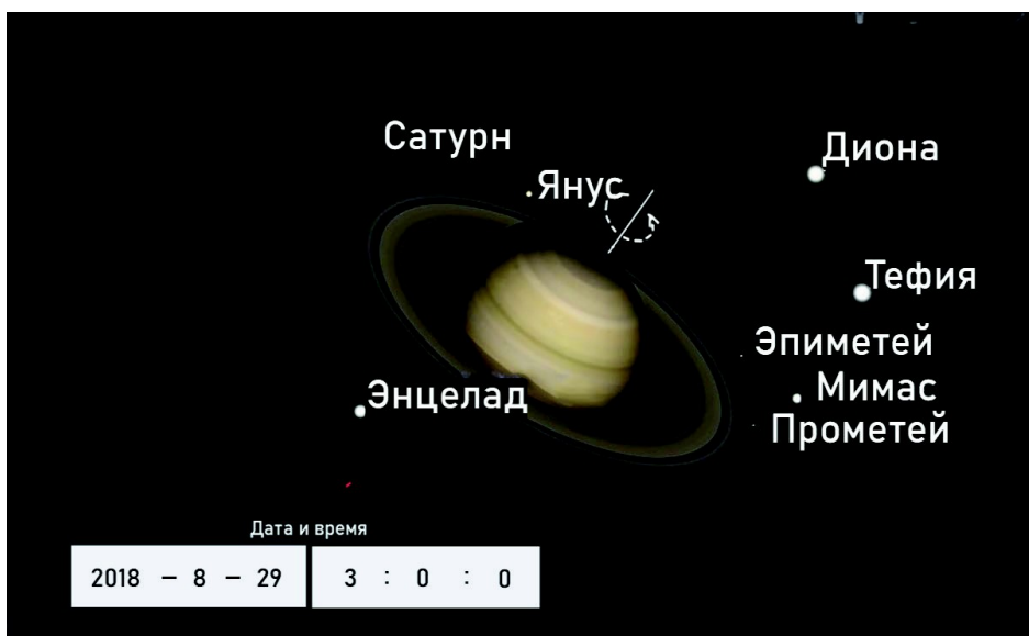
Рисунок 3-38. Раскрытие северного полюса Сатурна
