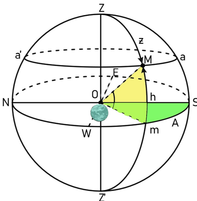
Рисунок 1-6. Система координат, тип которой необходимо определить
