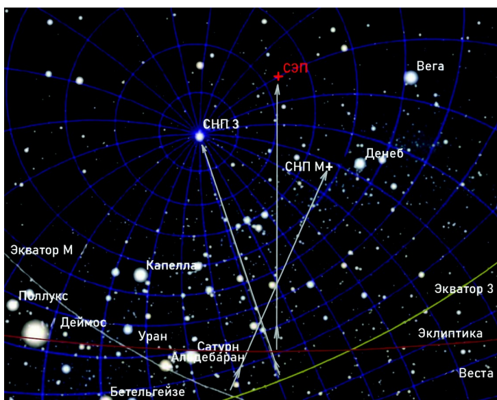
Рисунок 3-28. Расположение полюсов на небе Марса. Направления на полюсы на небесной сфере
