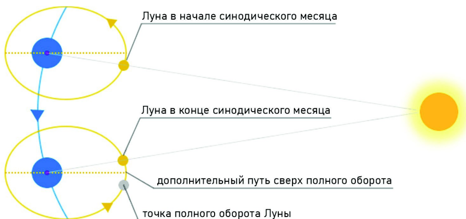
Рисунок 3-3. Схема, поясняющая различие синодического и сидерического периодов Луны
