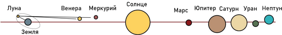
Углы наклона орбит планет Солнечной системы к плоскости эклиптики
