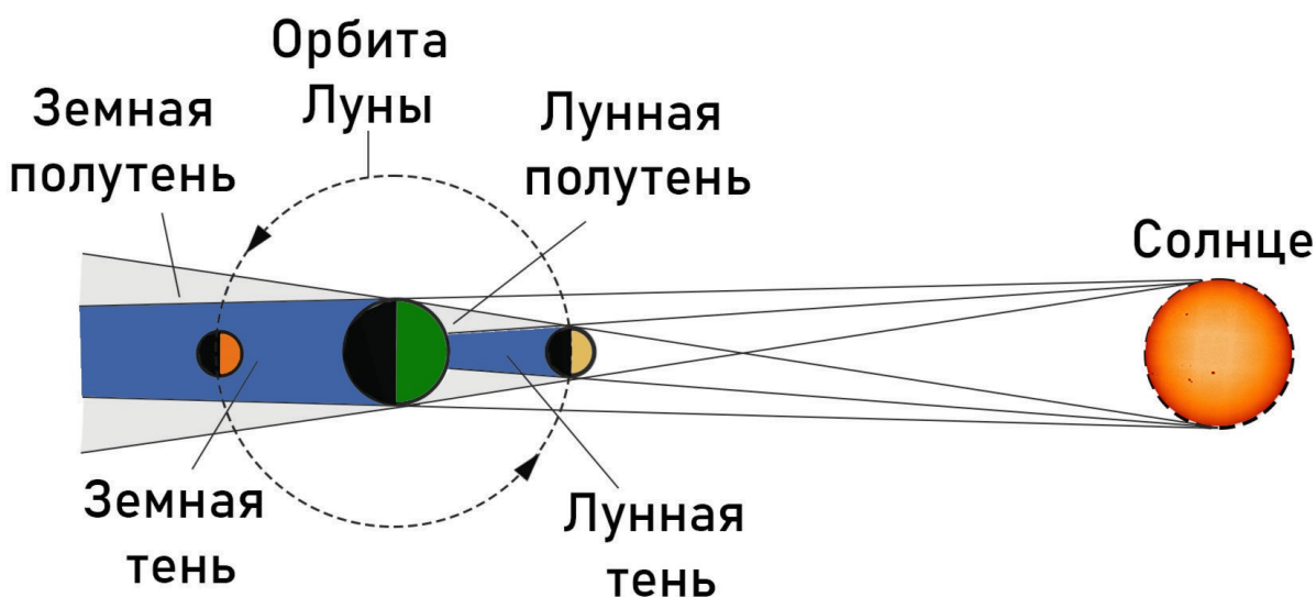
Рисунок 2-42. Схема получения затмений
