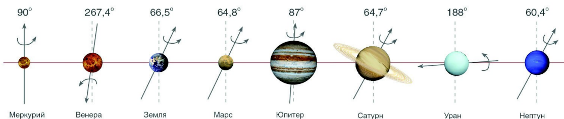
Рисунок 3-20. Наклон осей вращения планет к плоскости эклиптики
