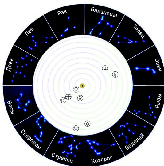
Рисунок Гл3-24. Расположение планет на дату 13.06.2001г
