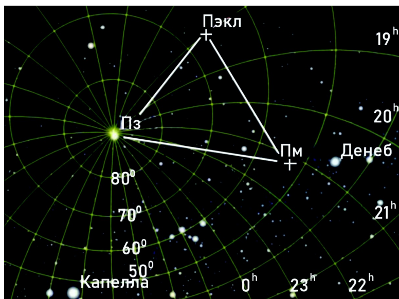
Рисунок 3-32. Полюс Земли в экваториальной системе Земли
