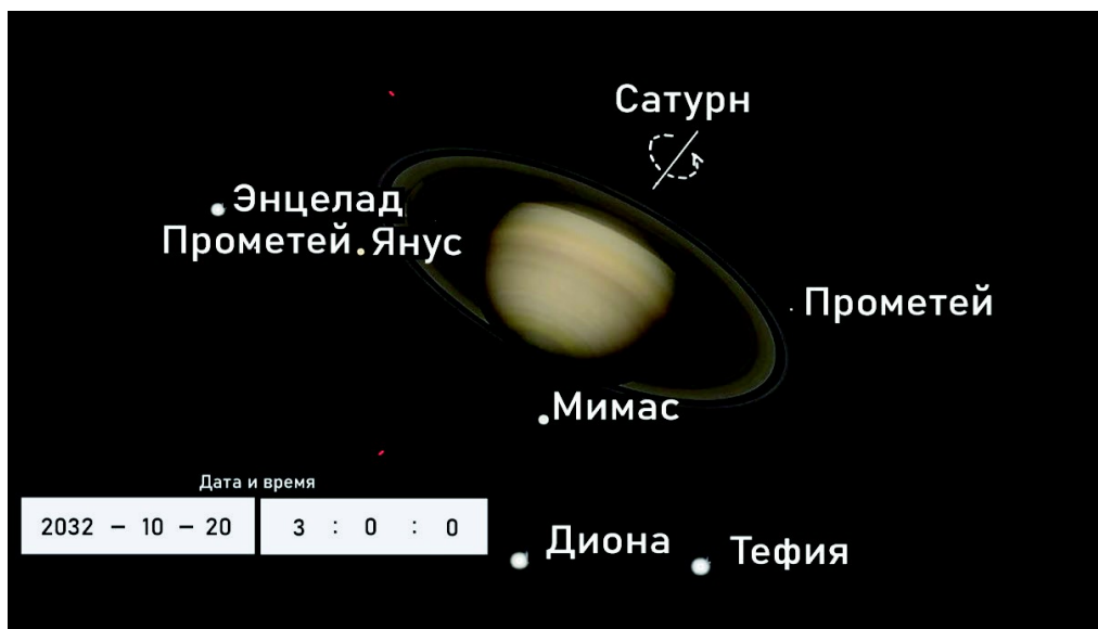
Рисунок 3-38. Раскрытие южного полюса Сатурна
