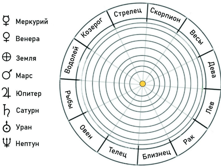
Рисунок 2-1 6. Шаблон орбит планет
