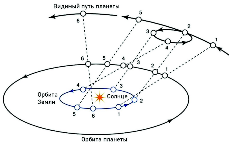
Рисунок 3-5. Схематическое изображение положения Земли и Марса
