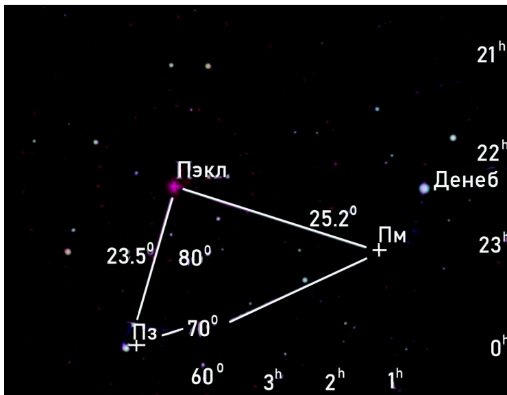
Рисунок 3-31. Полюс эклиптики в экваториальной системе Земли
